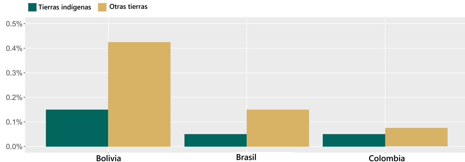
Tasas anuales de deforestación en Bolivia, Brasil y Colombia (2000- 2021)
